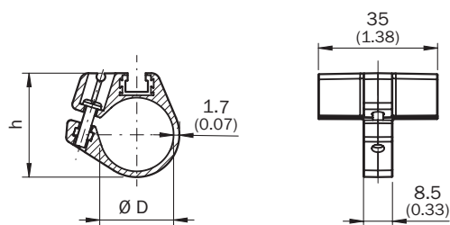
Размеры, мм
