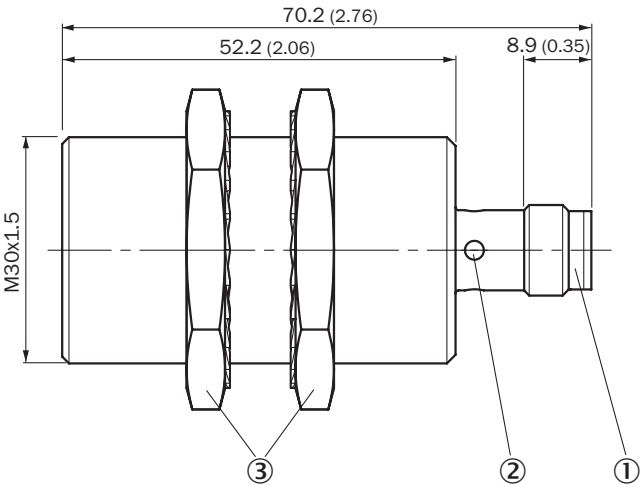
Габаритный чертёж IMB30 стандарт, штекер M12, вровень с плоскостью
