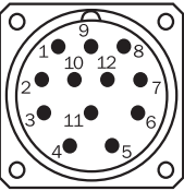
엔코더의 M23 수 장치 커넥터 보기
