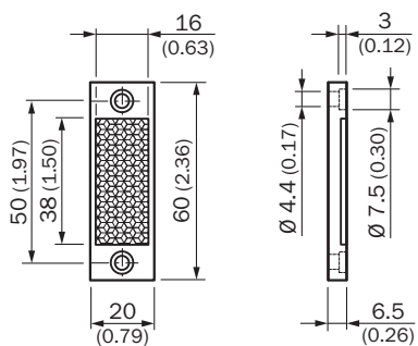
Размеры, мм
