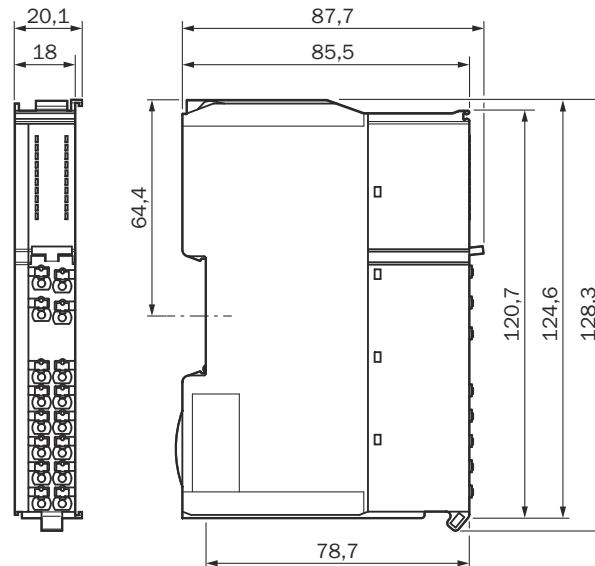
Illustration 15 : Plan coté
