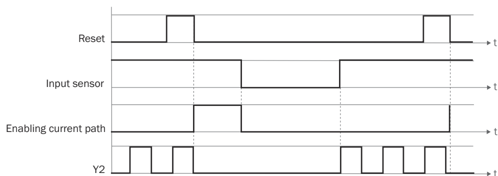
Illustration 4 : Déroulement/chronogramme
