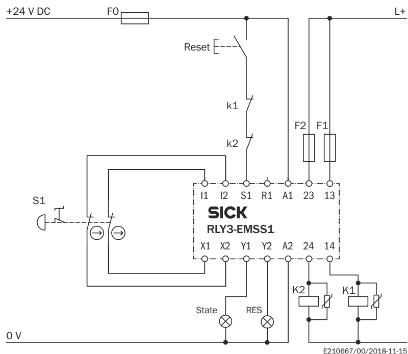
Illustration 5 : Exemple de câblage ReLy EMSS1, avec fonction de réarmement et contrôle des contacteurs commandés (EDM)
