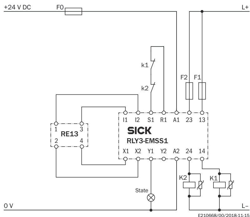
Illustration 6 : Exemple de câblage ReLy EMSS1, sans fonction de réarmement, avec contrôle des contacteurs commandés (EDM)
