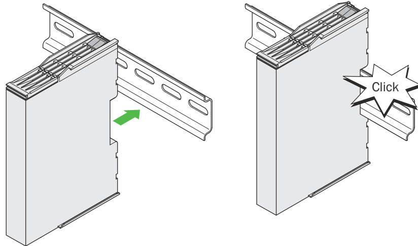
Illustration 7 : Montage
