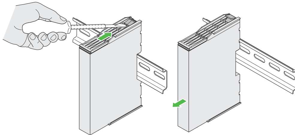
Illustration 9 : Démontage
