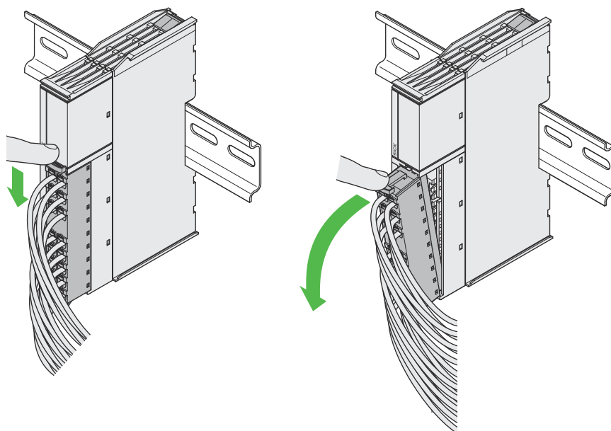
Illustration 10 : Démonter le connecteur frontal
