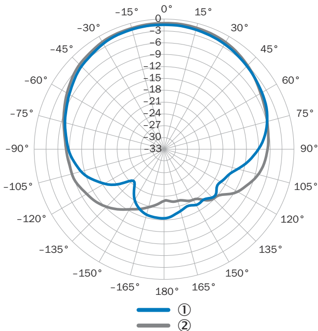
圖 3: RFU61x 整合式天線的方位圖 (典型值): 866.5 MHz 時所測的天線增益以 dBic 計, LHCP (左旋圓極化)
