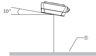
圖 2: 正面金屬面較大時選擇安裝角度，如 10°
