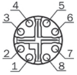
圖 6: M12 8-Pin 母接頭, X 型編碼
