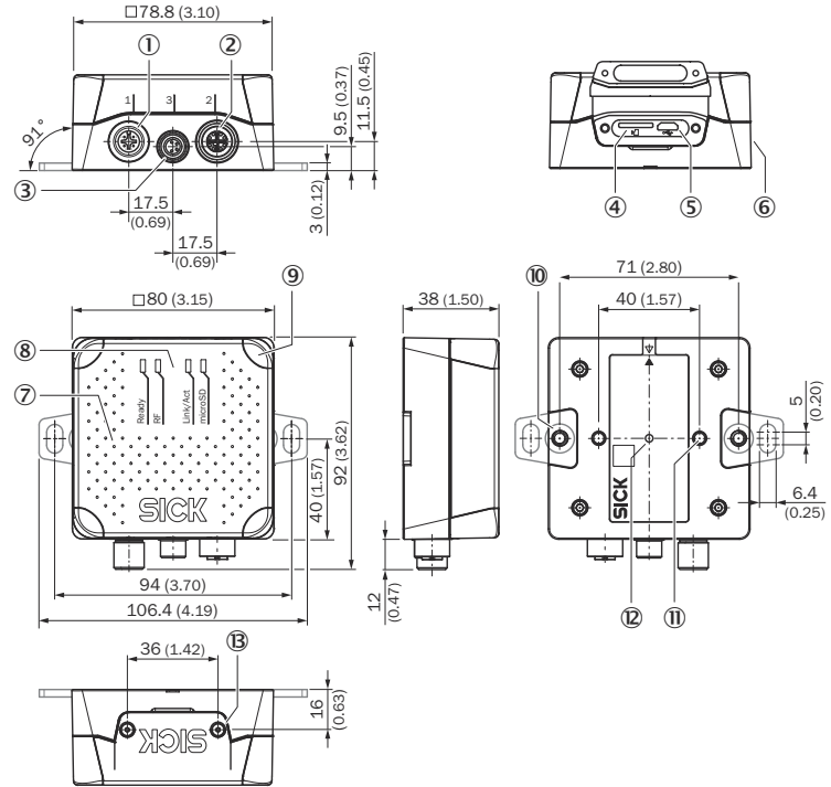
圖 1: RFU610-106xx 的尺寸圖，量測單位：mm (英吋)，小數分隔符：點
