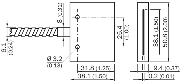
Maattekening LISR40900, LBSR40900
