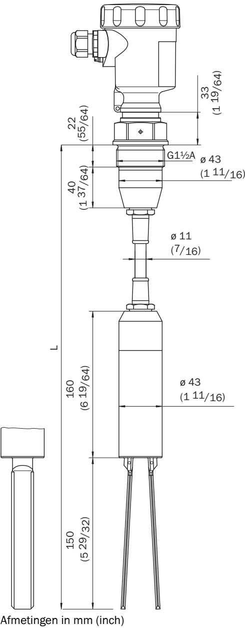
Maattekening LBV320 met PUR-draagkabel, schroefdraaduitvoering G 1½ A (DIN ISO 228/1)
