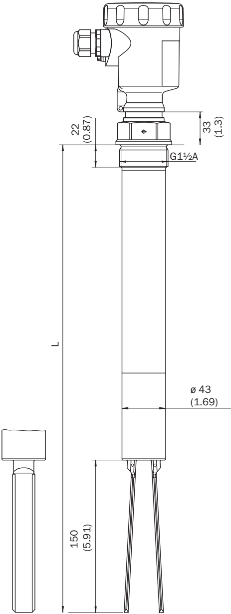
Maattekening LBV330 schroefdraaduitvoering G 1½ A (DIN ISO 228/1)
