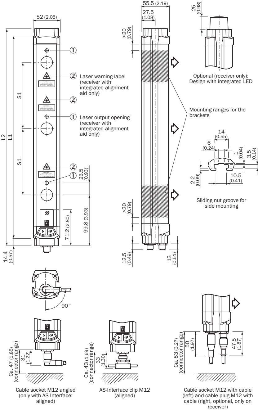
Afmetingen in mm (inch) Zender/ontvanger in één behuizing
