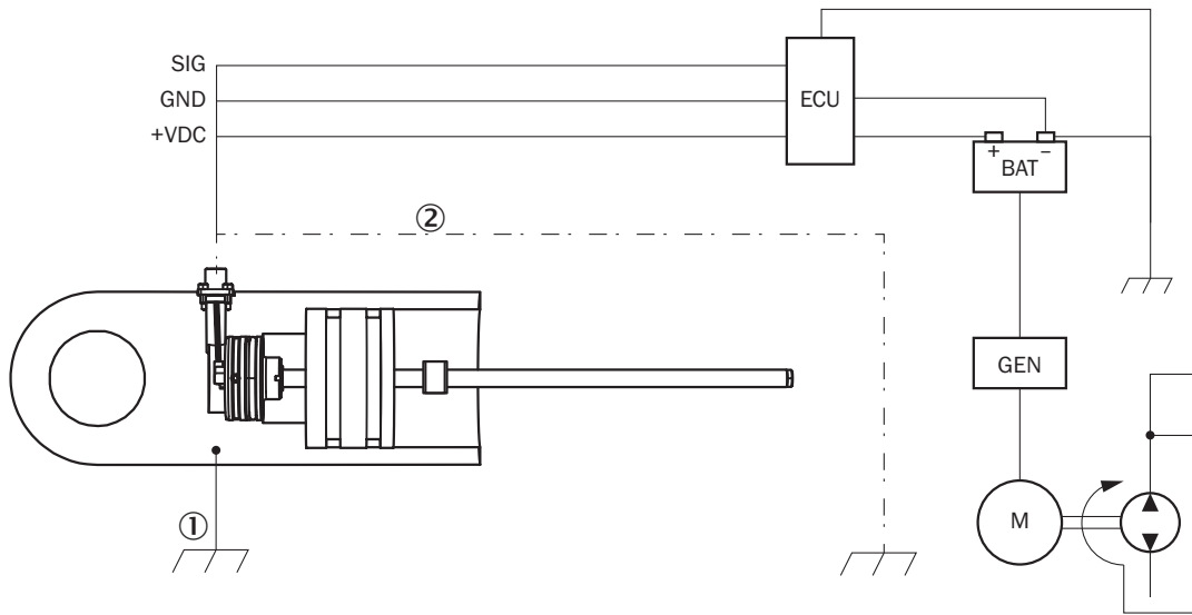
Aansluitschema
