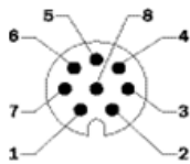
Ansicht Gerätestecker M12 an Leitung/Gehäuse
