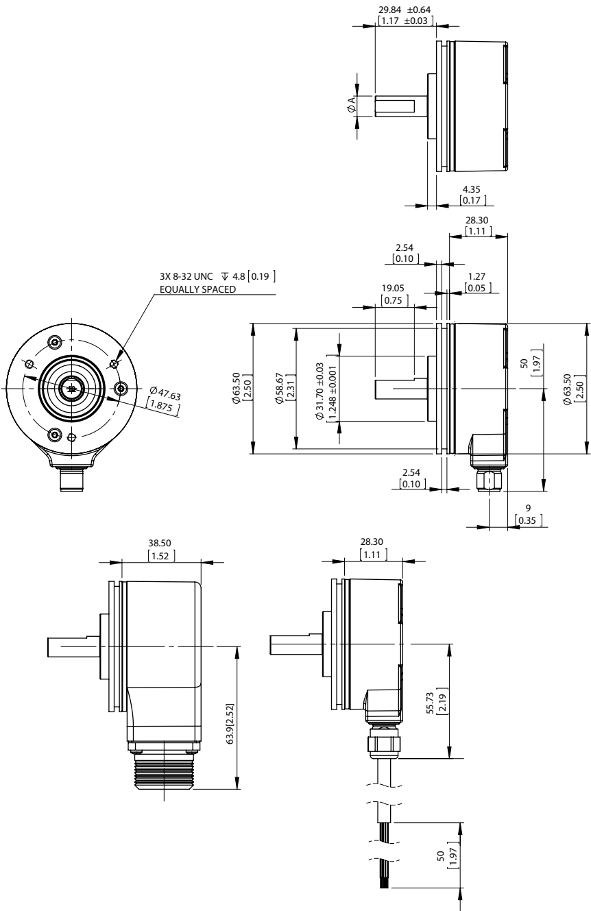
Maattekening DFS25 servoflens, radiale stekkeruitvoering M12 en MS, kabeluitgang
