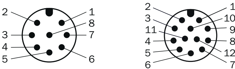
Aanzicht apparaatstekker M12 aan encoder
