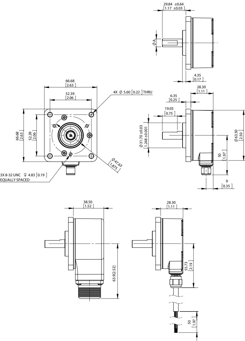
Maattekening DFS25 vierkante flens, radiale stekkeruitvoering M12 en MS, kabeluitgang
