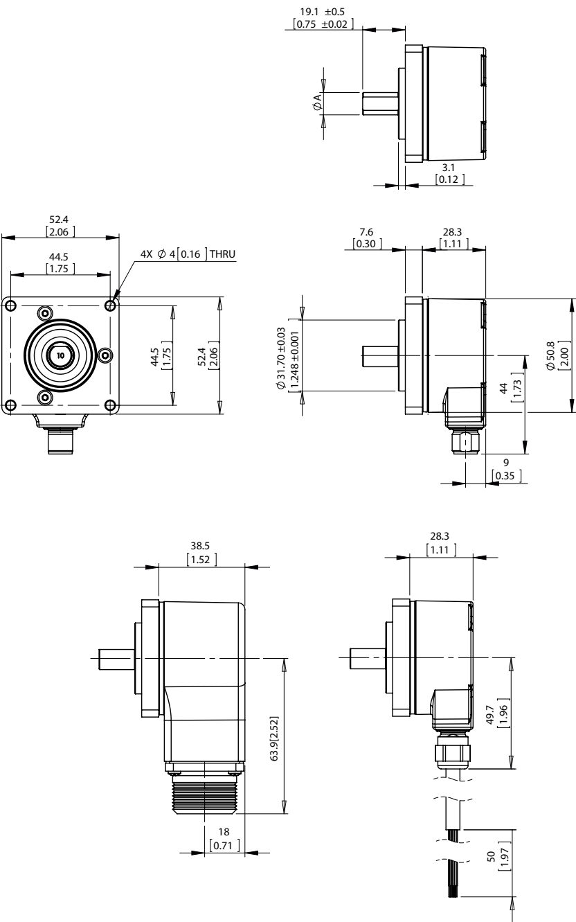
Maattekening DFS20 vierkante flens, radiale stekkeruitvoering M12 en MS, kabeluitgang
