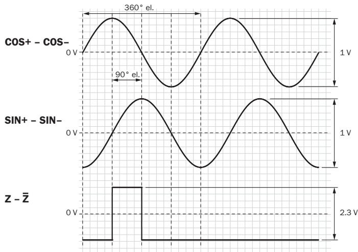
Bij draaiing van de as met de klok mee en blik in richting 'A' (zie maatschets)
