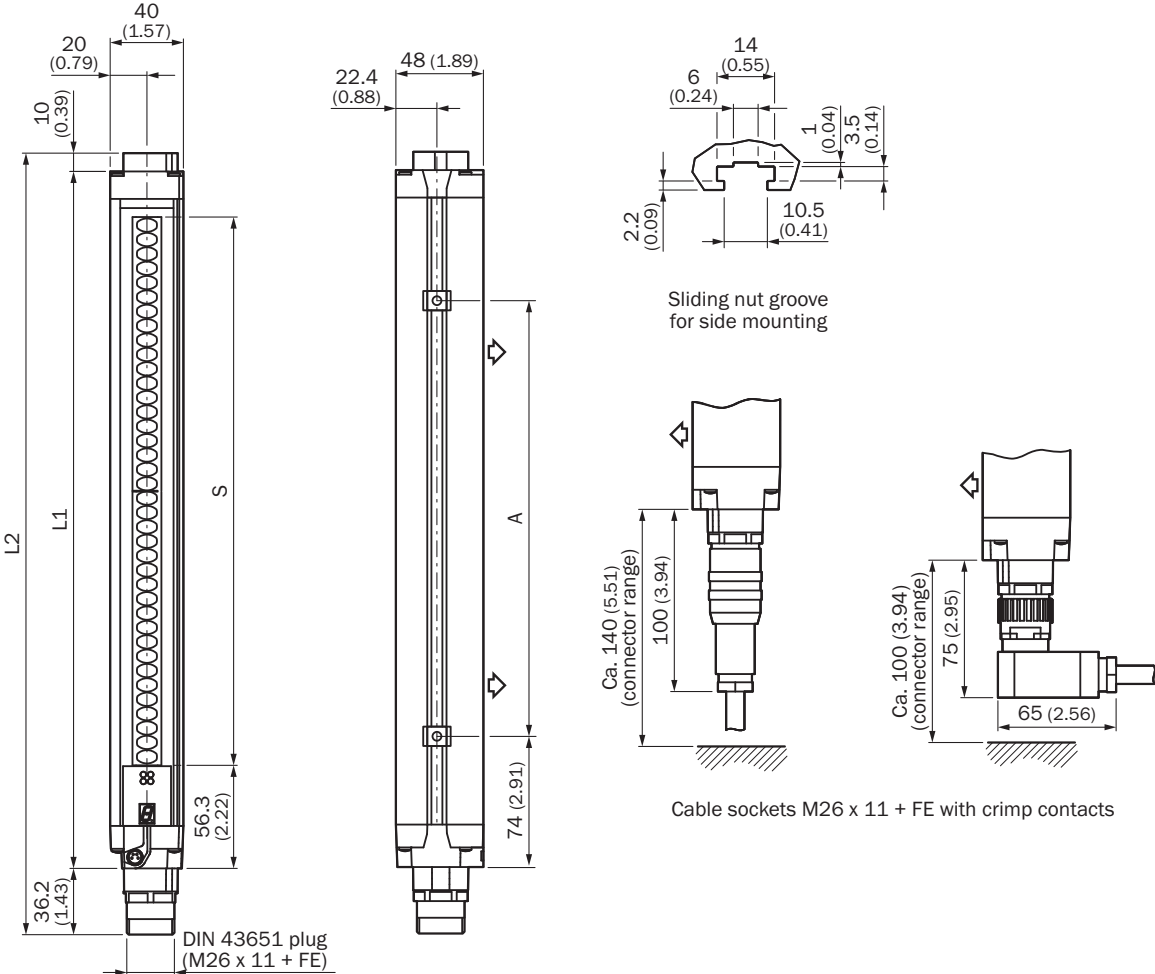
Afmetingen in mm (inch) Weergave zender (ontvanger in spiegelbeeld)
