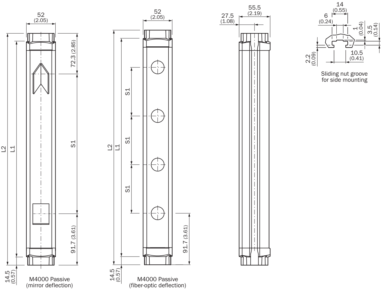
Afmetingen in mm (inch) omkeereenheid
