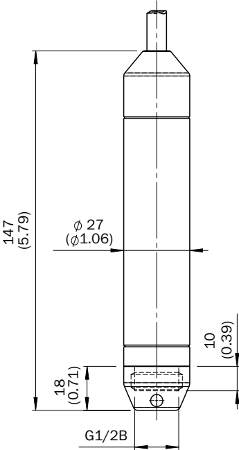
Dimensions en mm (inch)
