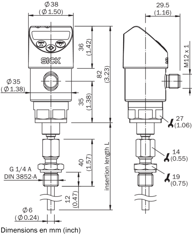
Plan coté Raccord de serrage à vis G ¼ A
