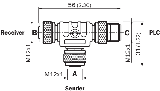
Plan coté SBO-02F12-SM
