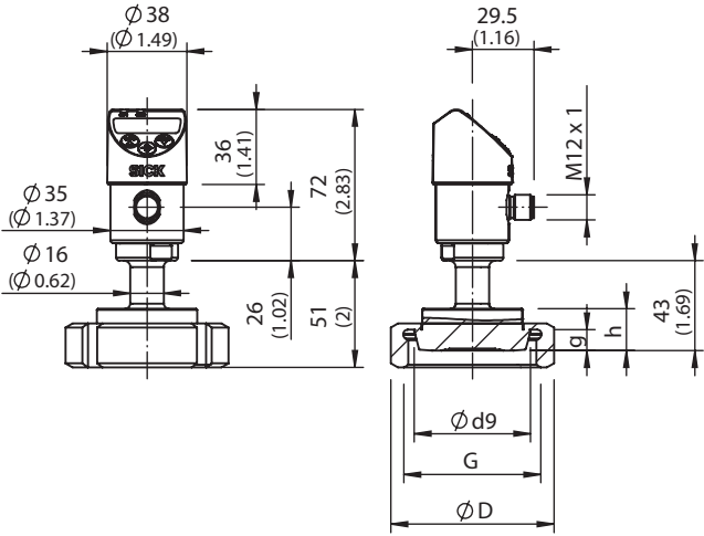
Plan coté Embout conique (DIN 11851) avec écrou à chapeau rainuré
