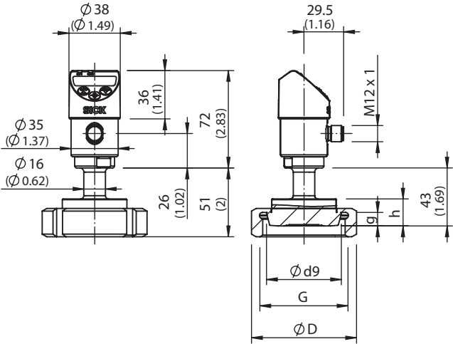
Plan coté Embout conique (DIN 11851) avec écrou à chapeau rainuré
