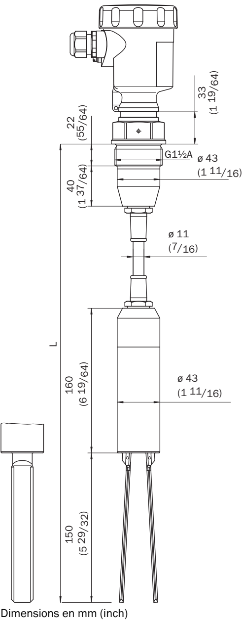
Plan coté LBV320 avec câble porteur PUR, version à filetage G 1½ A (DIN ISO 228/1)
