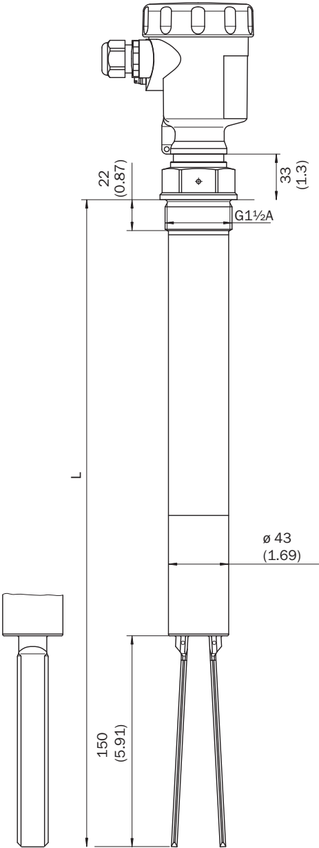
Dimensions en mm (inch)
