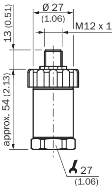
Dimensions en mm (inch)
