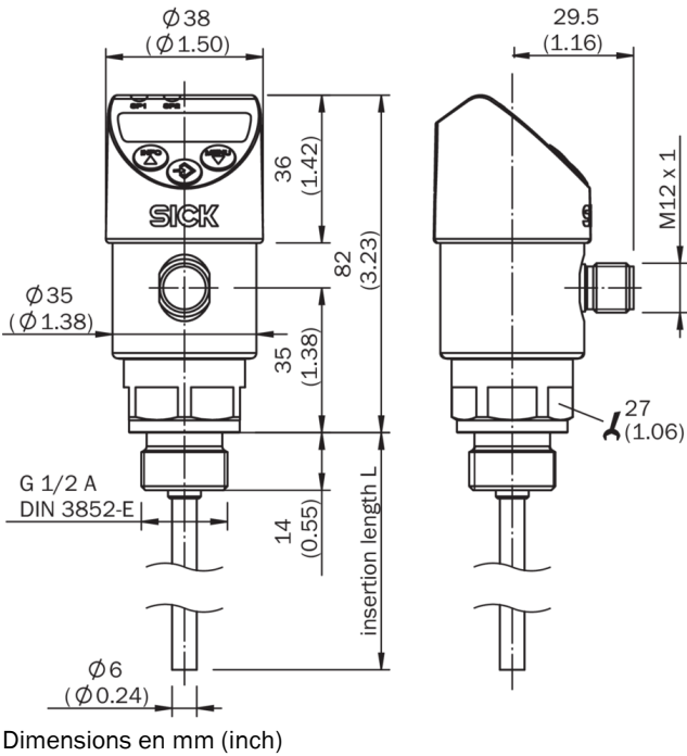
Plan coté TBS avec raccordement F <math>\frac{1}{2}</math> A selon DIN 3852-E
