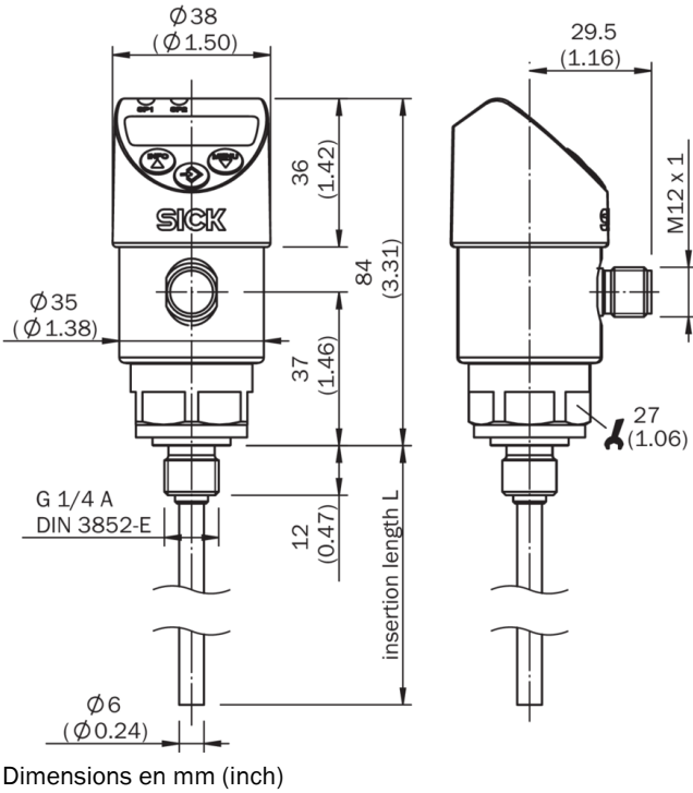
Plan coté TBS avec raccordement F 1/4 A selon DIN 3852-E
