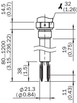
Dimensions en mm (inch)
