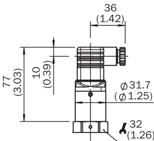
Dimensions en mm (inch)
