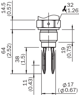
Dimensions en mm (inch)
