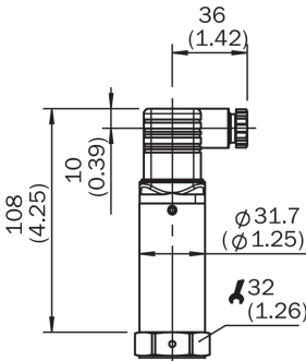
Dimensions en mm (inch)
