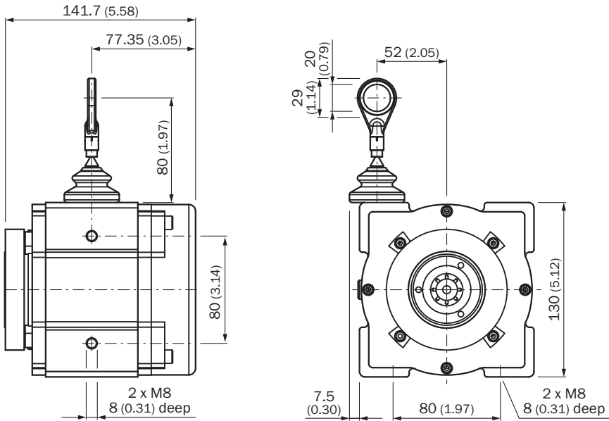
Dimensions en mm (inch)
