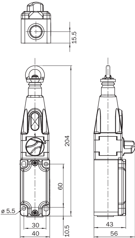
Dimensions en mm (inch)
