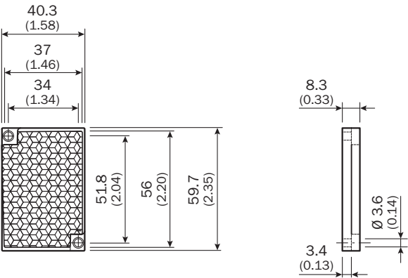
Dimensions en mm (inch)
