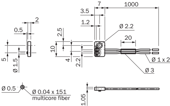
Plan coté LL3-DE01
