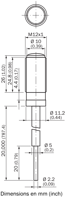
Plan coté LL3-TX02
