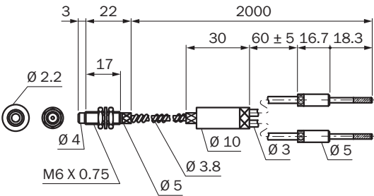
Plan coté LL3-DH03
