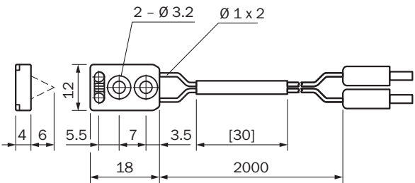
Plan coté LL3-DC38
