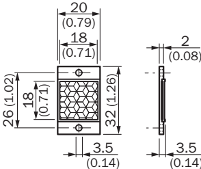
Dimensions en mm (inch)
