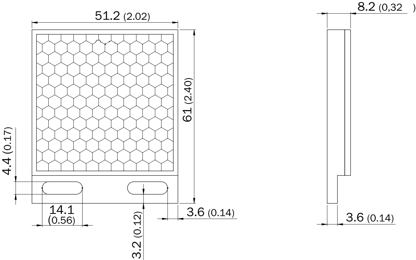
Dimensions en mm (inch)
