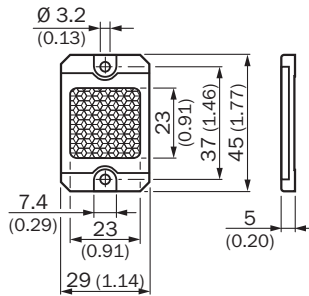
Dimensions en mm (inch)
