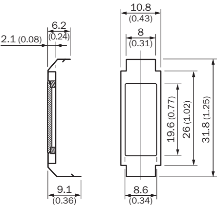
Dimensions en mm (inch)
