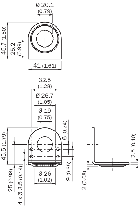
Dimensions en mm (inch)
