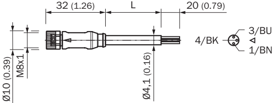
Dimensions en mm (inch)
