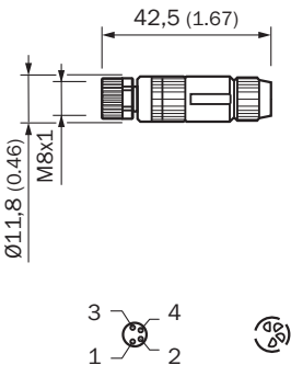
Dimensions en mm (inch)
