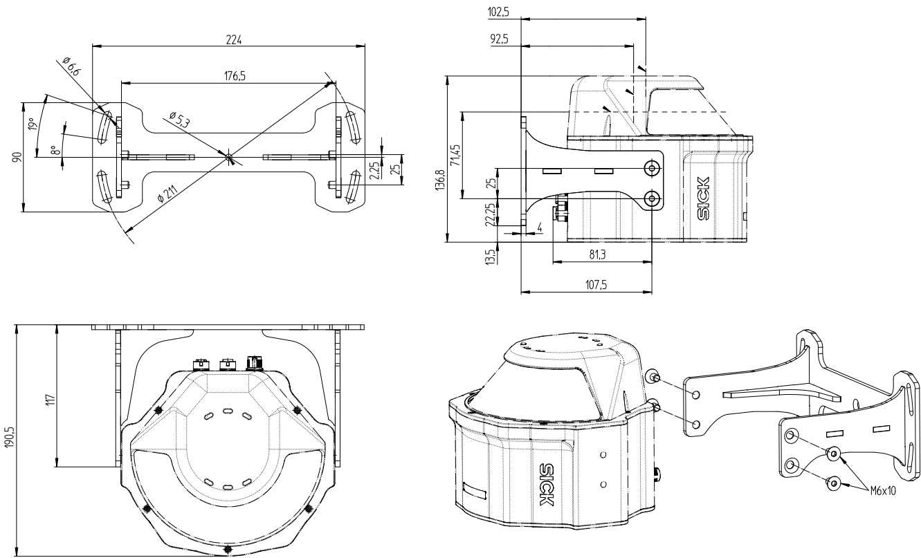
Dimensions en mm (inch)
