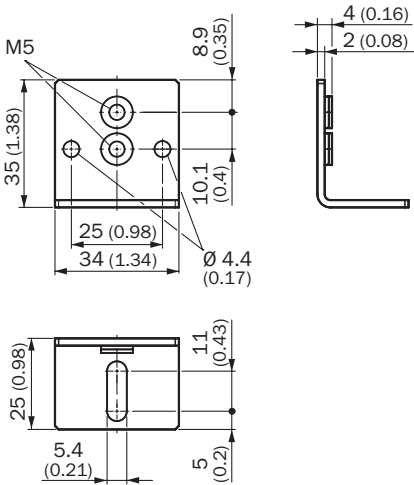
Dimensions en mm (inch)
