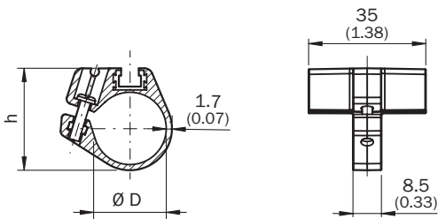
Dimensions en mm (inch)
