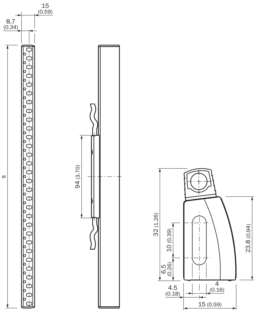
Dimensions en mm (inch) S = champ de protection = longueur du boîtier
