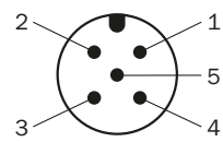
Connecteur mâle M12, 5 pôles, codage A
